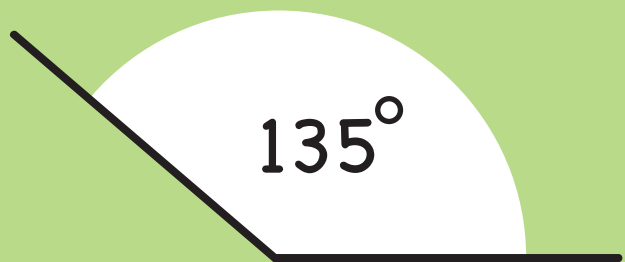
stumpfer Winkel
